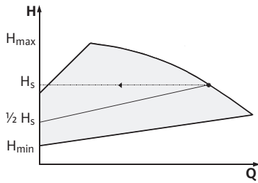
Fig.16: Регулирование Др-ν
