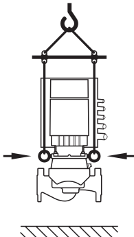
Fig. 8: Транспортировка насоса
