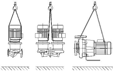
рис. 4: Строповка насоса
