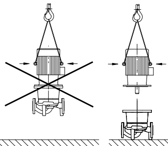
рис. 5: Строповка мотора
